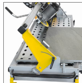
45 Grad-Schnitte von der rechten Seite. Der Seitentisch kann einfach ohne Werkzeuge links und rechts fixiert werden.
